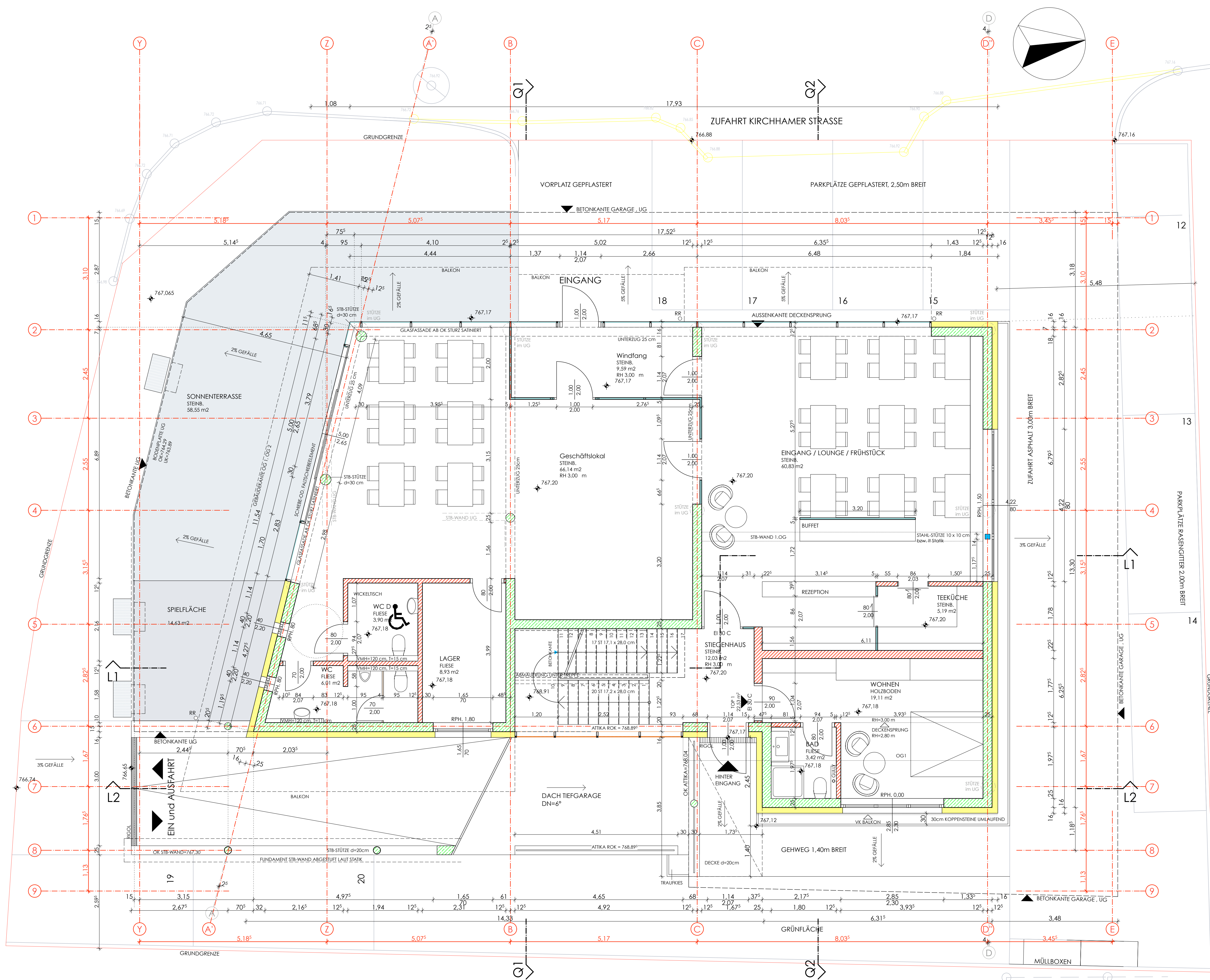
GRUNDRISS ERDGESCHOSS 1:50
